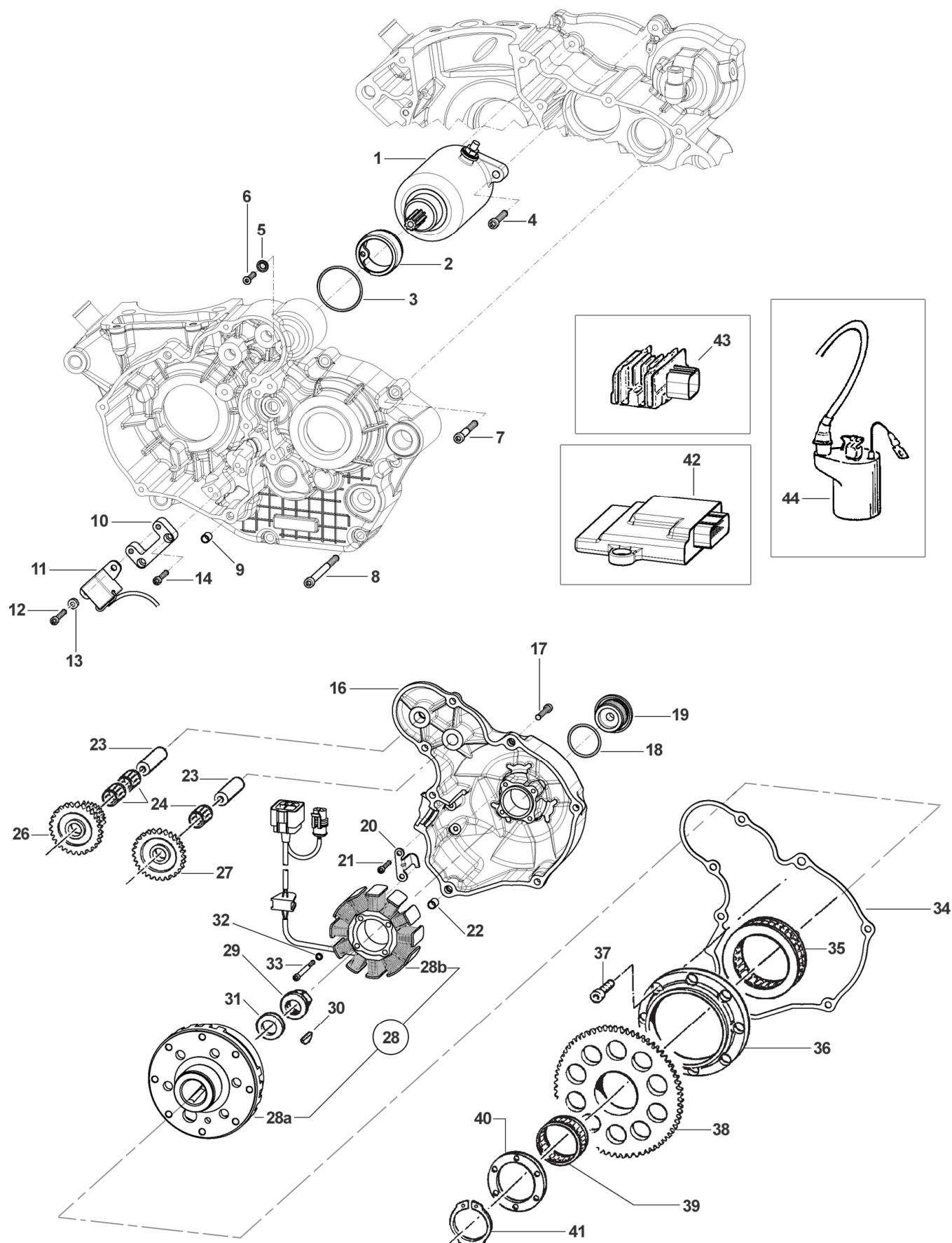
Tav. 10 – Avviamento Elettrico + Generatore E.S. MX/SMX con batteria (Electric starter + generator E.S. MX/SMX with battery)
